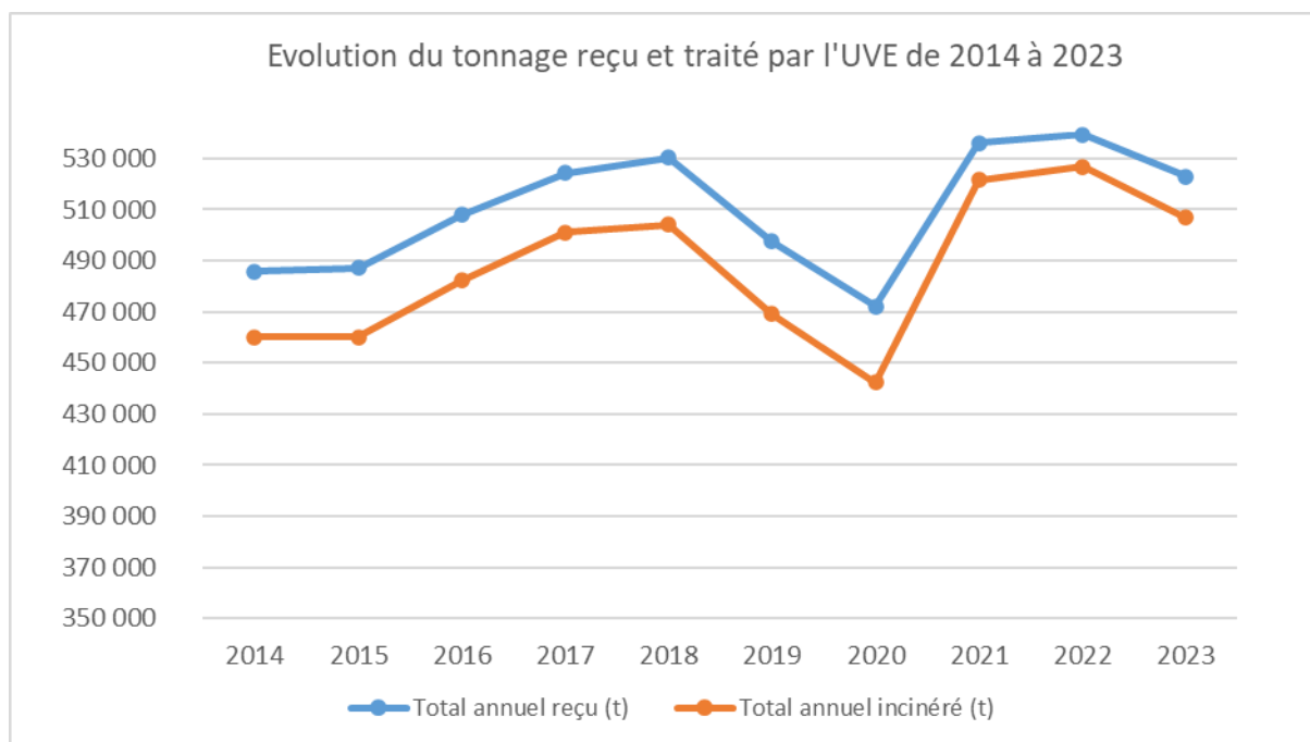
Figure 12 : Graphique des tonnages annuels d'OM reçus et incinérés de 2014 à 2023
