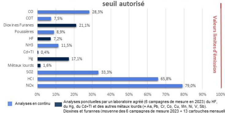
Figure 1 : Feuille de synthèse de l'activité 2023 d'Isséane
