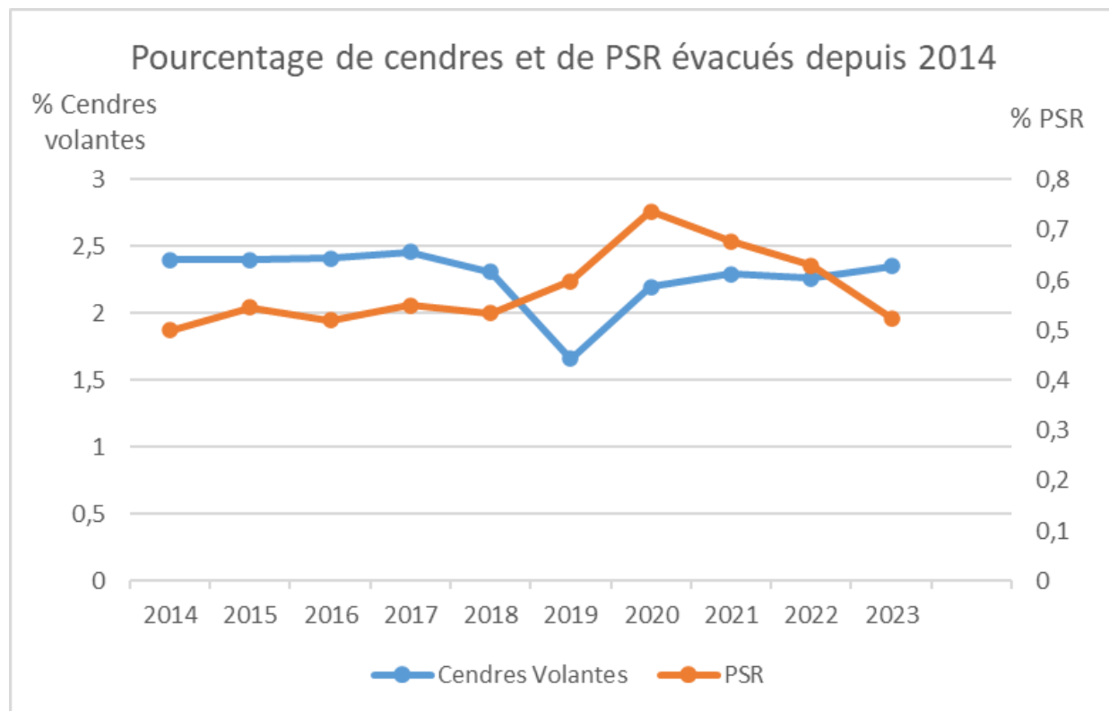
Figure 19 : Historique du pourcentage de cendres et PSR par rapport au tonnage incinéré depuis 2014
