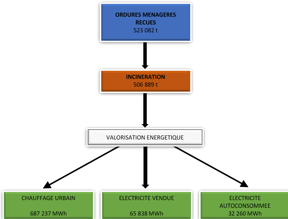
Figure 20 : Schéma du bilan énergétique de l'UVE en 2023
