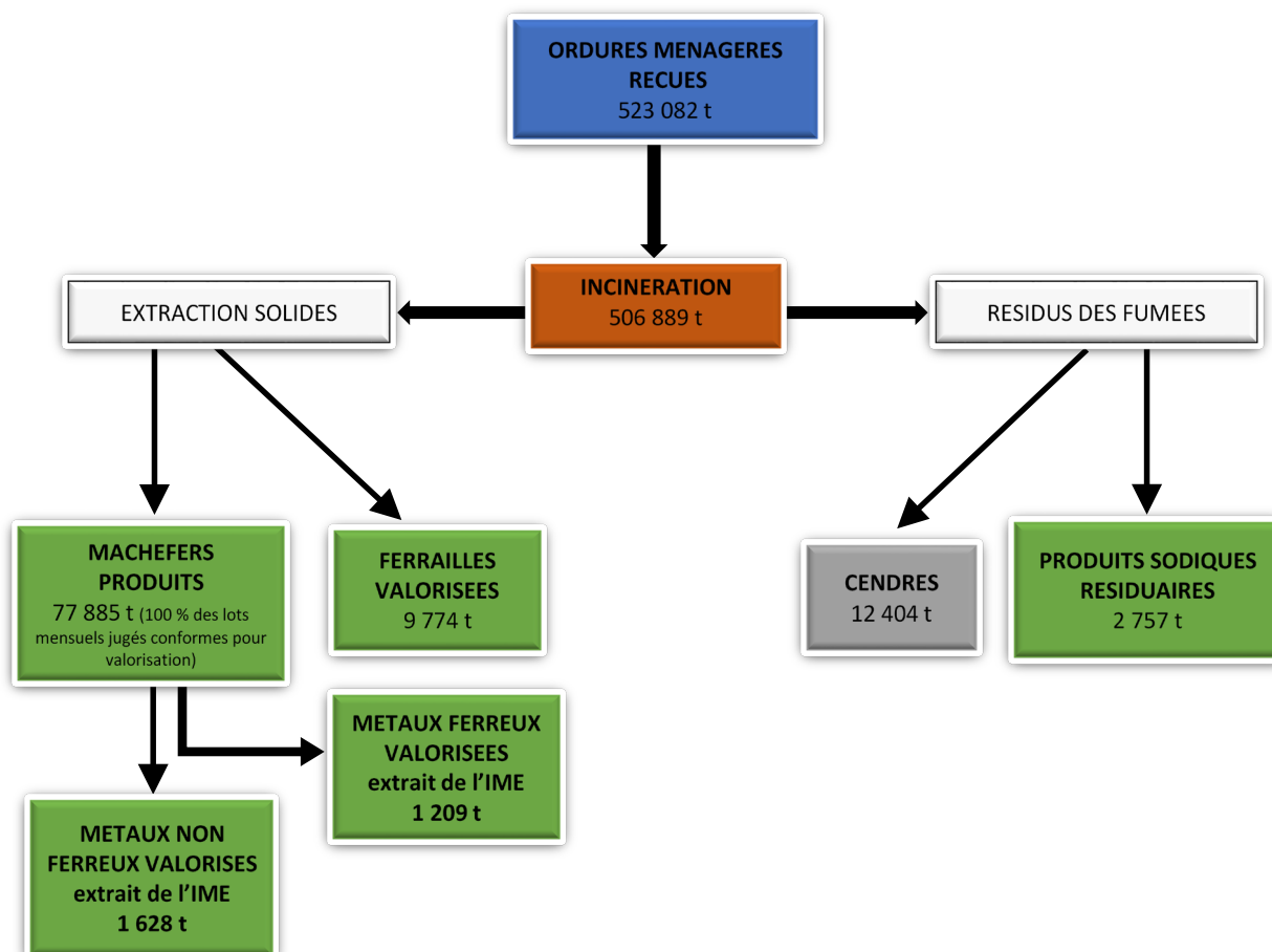
Figure 15 : Schéma du bilan matière de l'UVE en 2023 2
