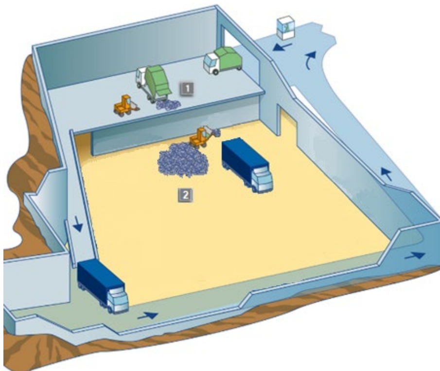
Figure 4 : Schéma du Centre de transfert
