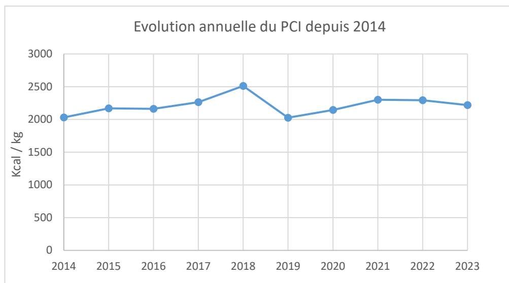
Figure 13 : Graphique de l'évolution annuelle du Pouvoir Calorifique Inférieur (kcal/kg) depuis 2014 pour l'UVE
